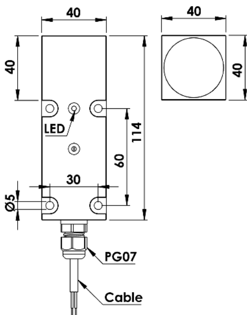
ابعاد سنسور
