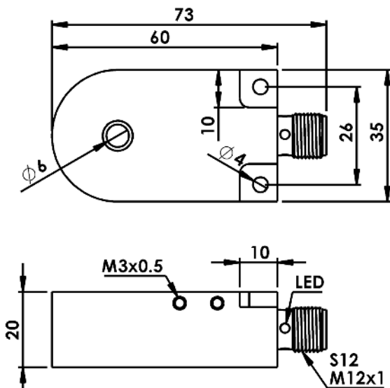
ابعاد سنسور
