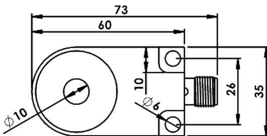
ابعاد سنسور
