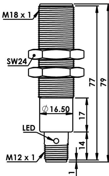
ابعاد سنسور
