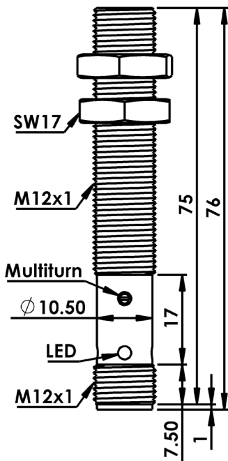
ابعاد سنسور
