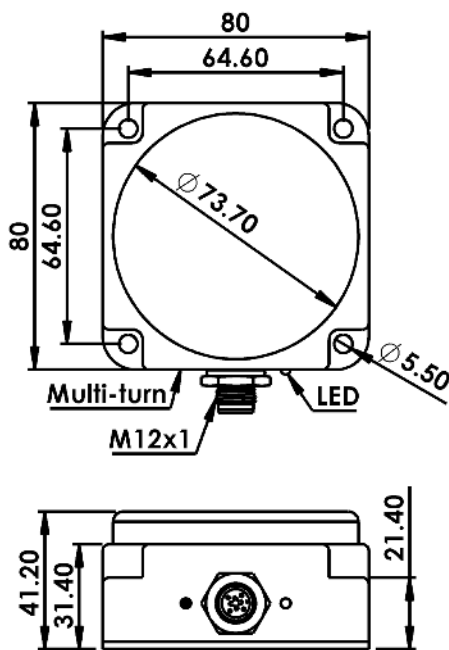
ابعاد سنسور
