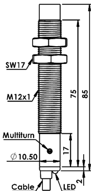
ابعاد سنسور
