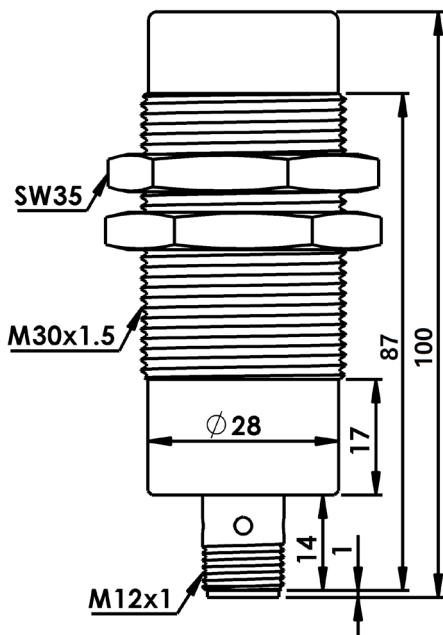
ابعاد سنسور
