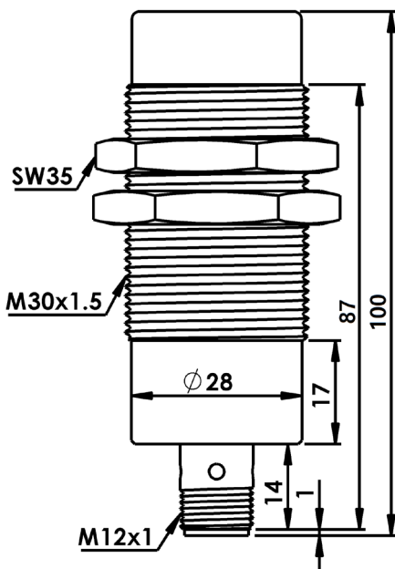
ابعاد سنسور
