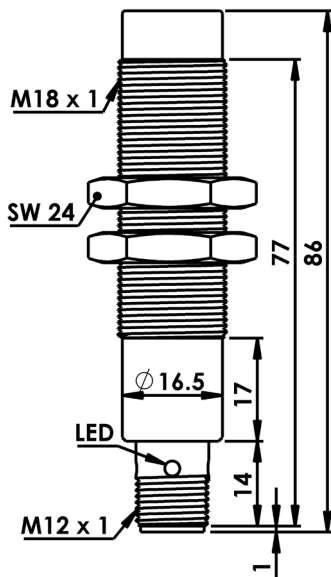
ابعاد سنسور
