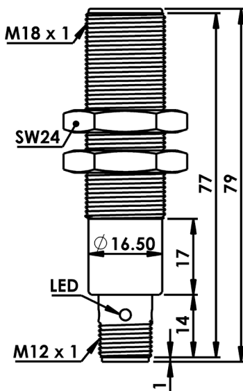
ابعاد سنسور
