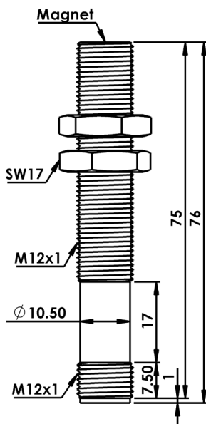
ابعاد سنسور
